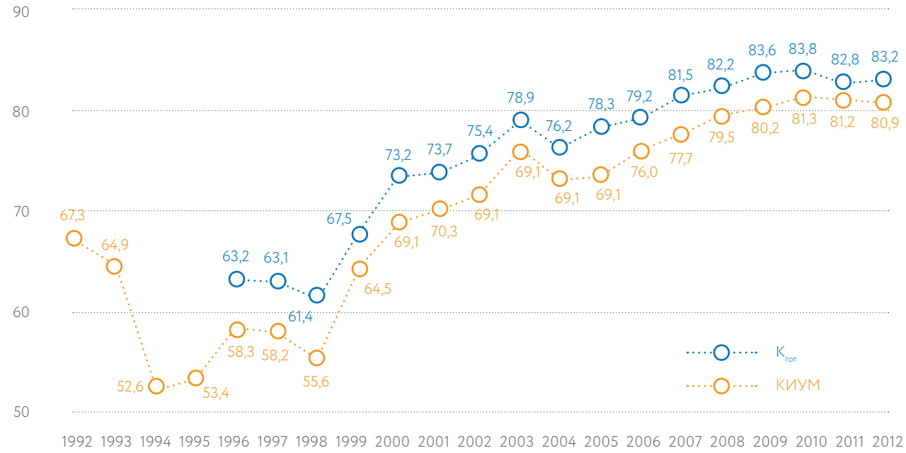
Коэффициент использования установленной мощности (КИУМ) и коэффициент готовности ( K_{\text{гот}} ) в динамике, %
