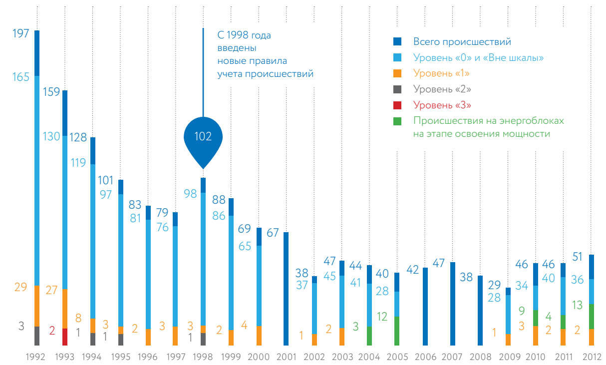
Количество происшествий по шкале INES на энергоблоках, находящихся в промышленной эксплуатации (в динамике)
