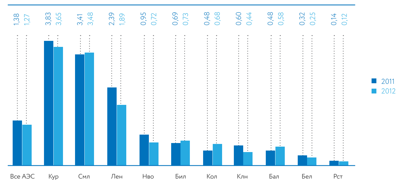
Коллективные дозы облучения на АЭС в 2011–2012 годах, чел.Зв/блок
