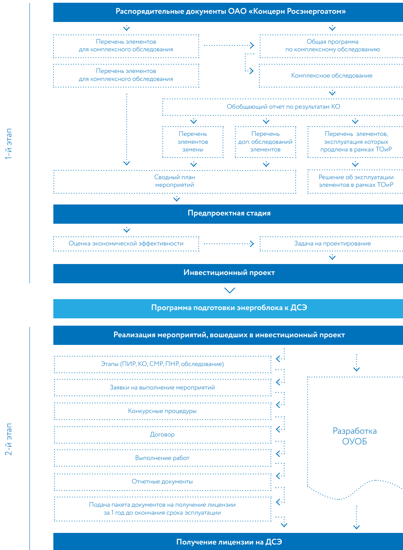
Схема управления продлением срока эксплуатации энергоблоков АЭС
