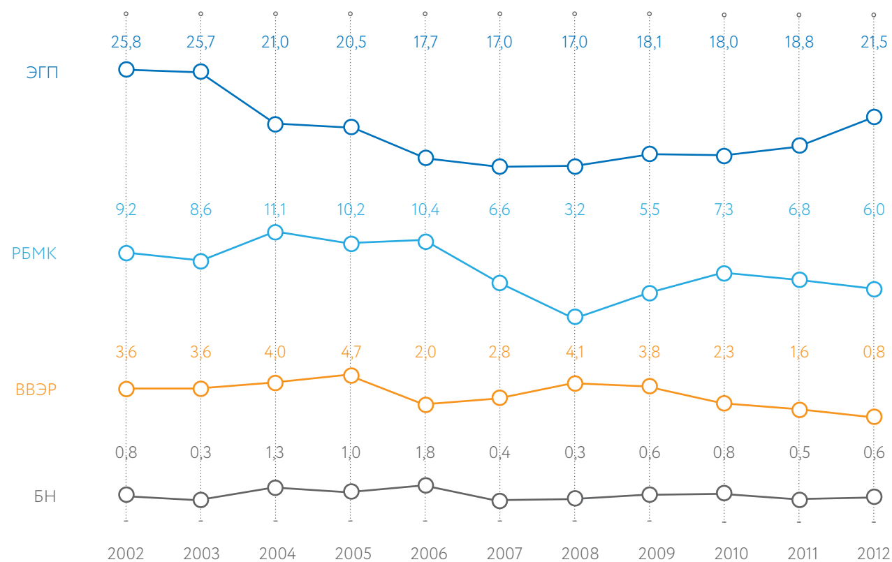
Выбросы инертных радиоактивных газов, в % допустимых выбросов
